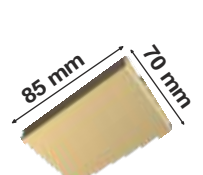
Τάπα τραβέρας 1504
