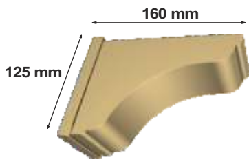
Τελείωμα τραβέρας 1502
