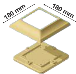
Πέλμα κολώνας 1500
